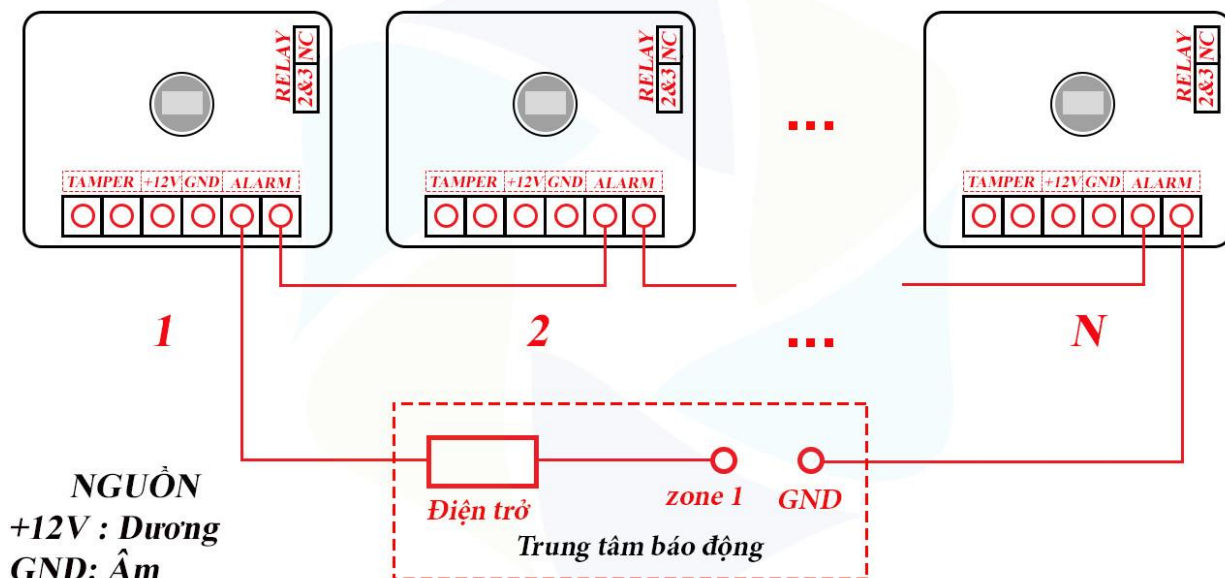
SƠ ĐỒ ĐẦU DÂY THƯỜNG ĐÓNG (NC) CHO HỒNG NGOẠI
